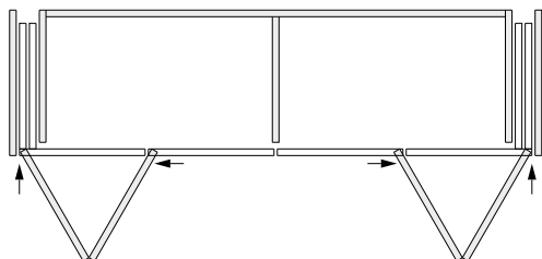
Hawa Folding Concepta III 20 Push, à gauche/à droite Aluminium, anodisé
