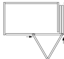
Hawa Folding Concepta III 20 Push, à droite Aluminium, anodisé
