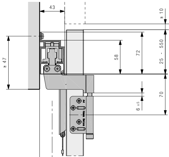
Rail de roulement montage mural
