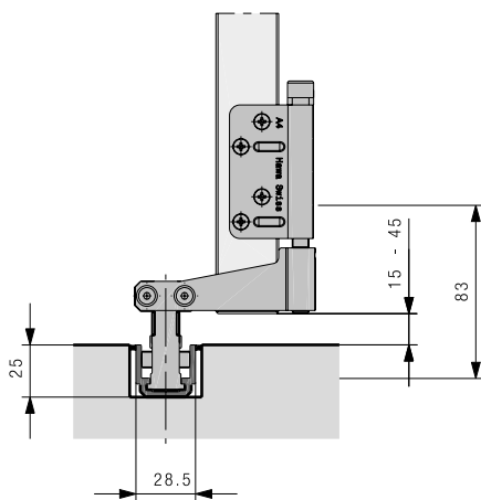
Rail de guidage intégré dans le sol
