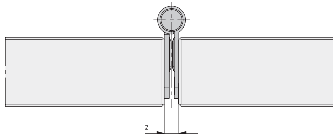
Variante 2, paumelle coudée : Z = 6mm
